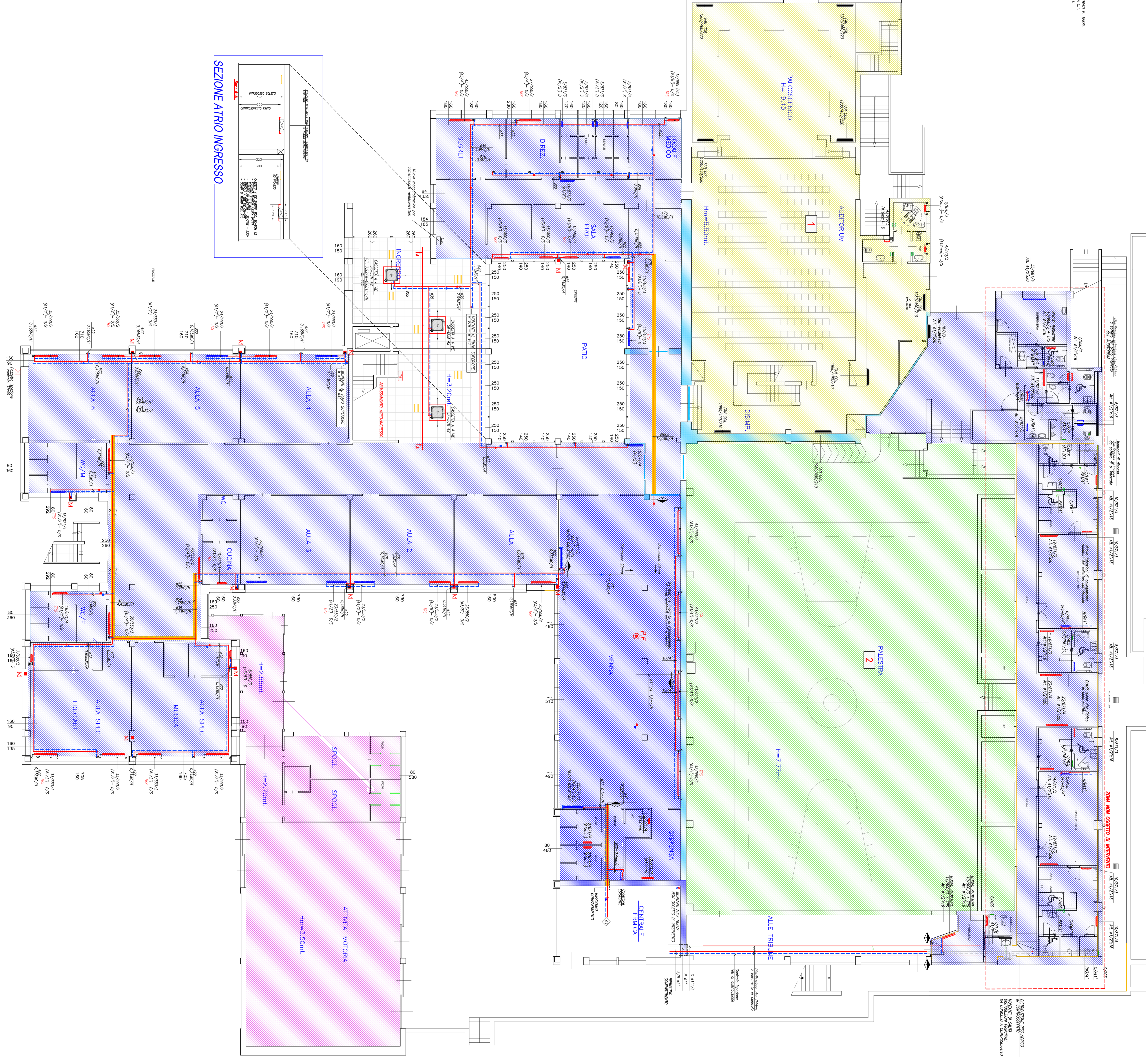
PIANTA PIANO TERRA
